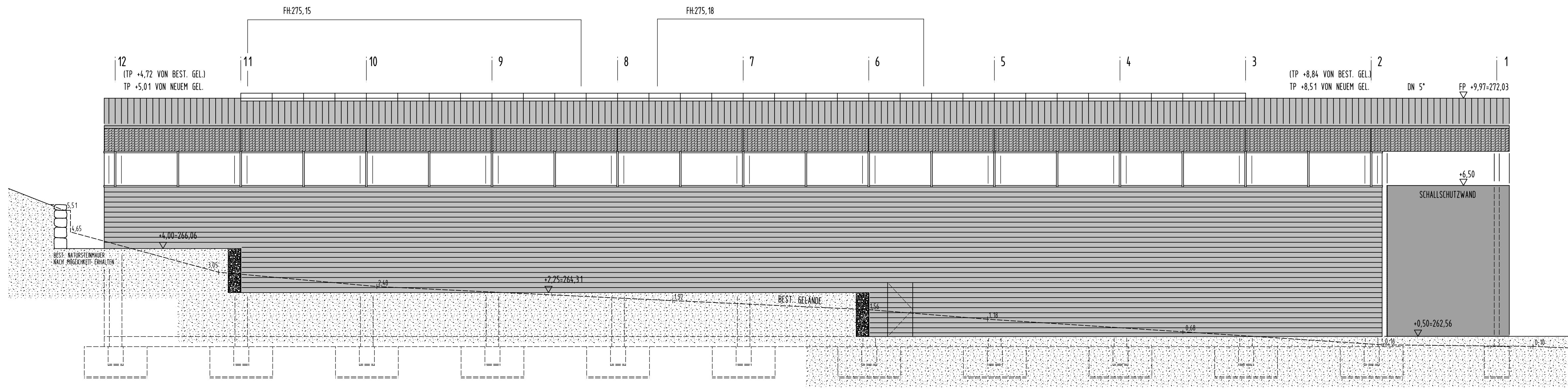
ANSICHT NORDWEST
