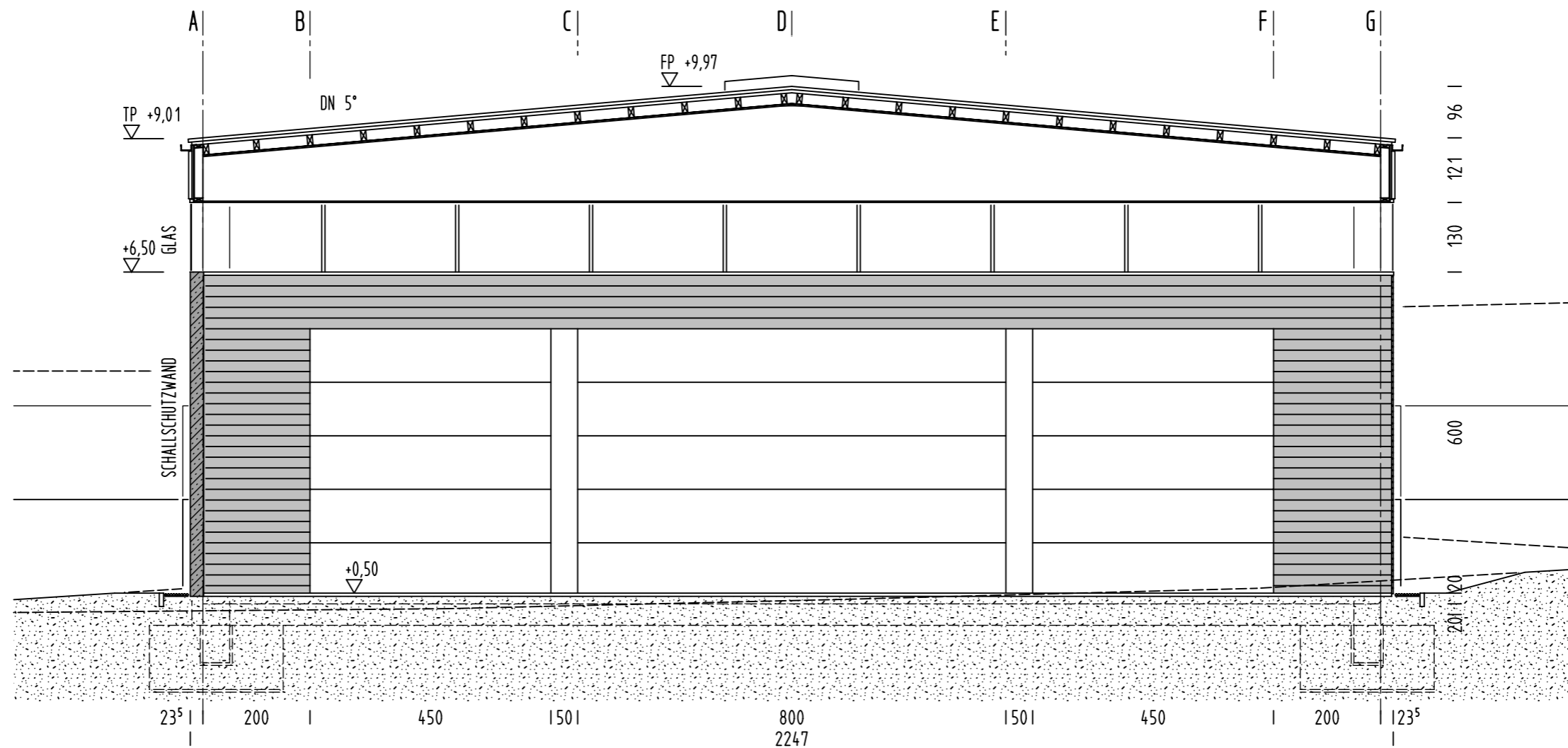
SCHNITT A-A
