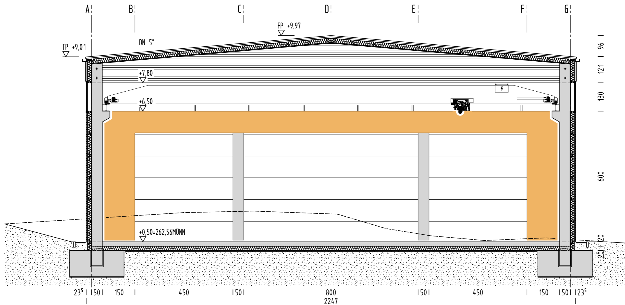
SCHNITT B-B
