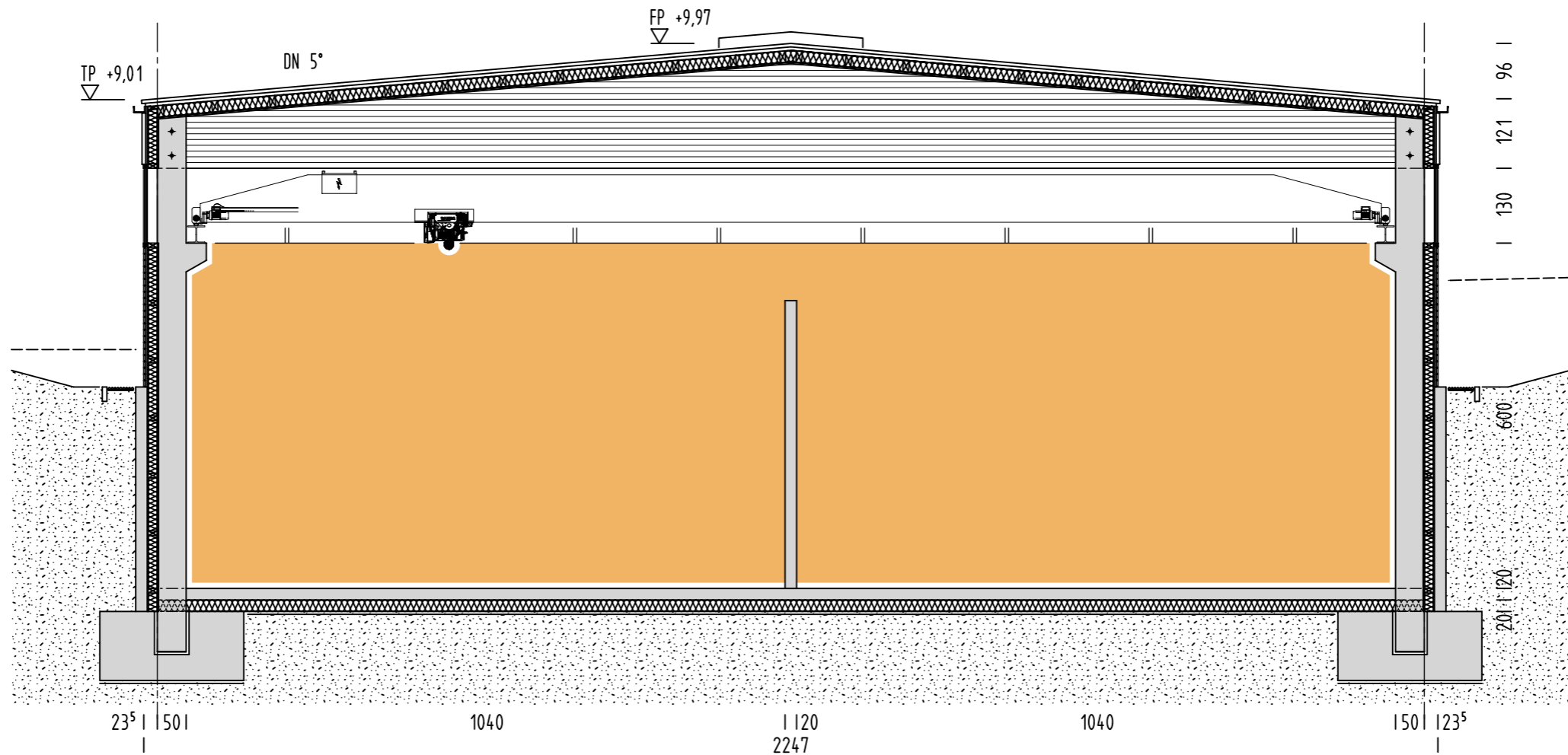
SCHNITT C-C
